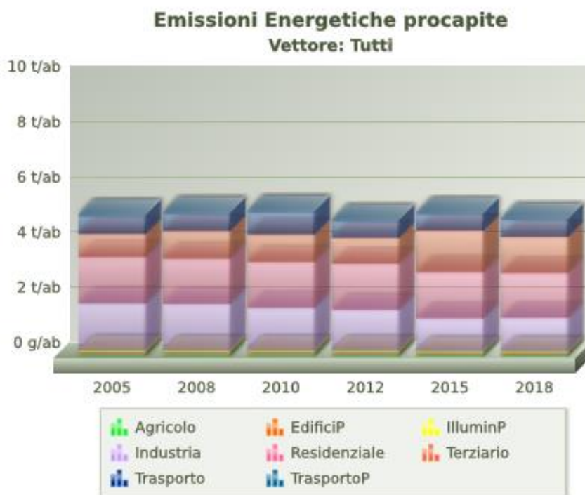
figura 3-4 _ trend delle emissioni di CO 2 comunali tra il 2005 e il 2018 ripartizione per settore (fonte: CO 20 )
