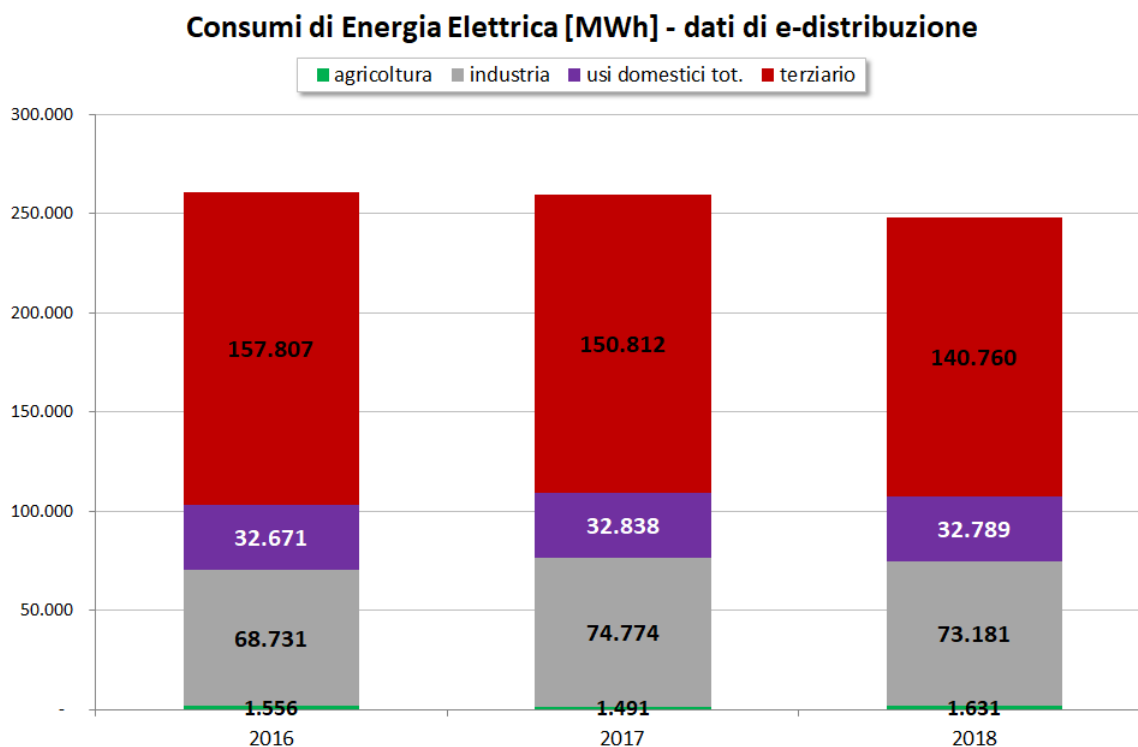
figura 3-1 _ consumi di energia elettrica dall'anno 2016 all'anno 2018 suddivisi per settore (fonte: E-distribuzione)
